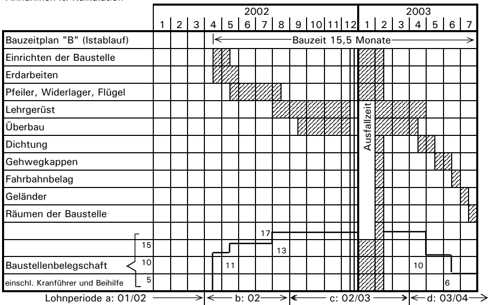
Korrektur Jahreszahlen und Lohnperioden Abb. D 4.5: Längsschnitt und Bauzeitenpläne
